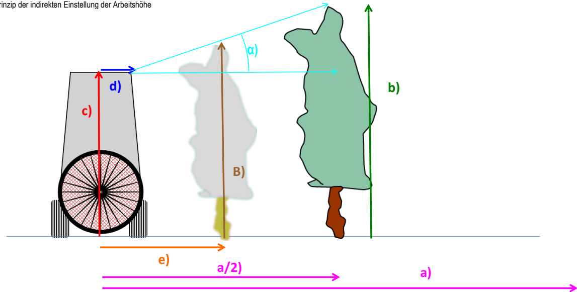
Prinzip der indirekten Einstellung der Arbeitshöhe
